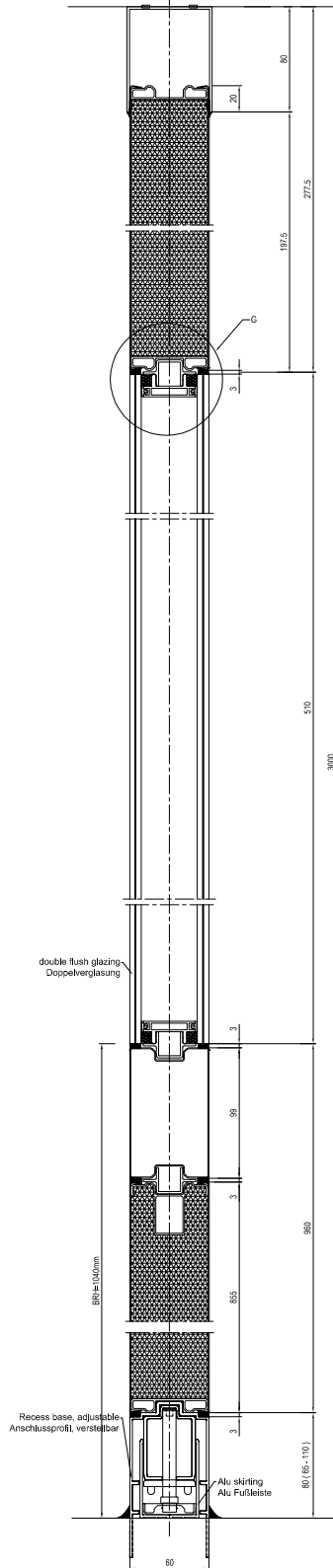
Trennwand mit Medienkanal Wall with media channel
