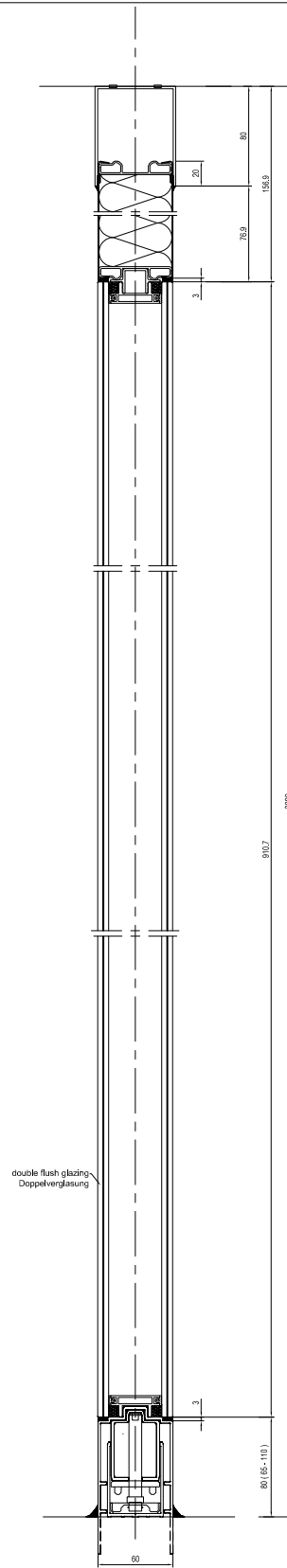
Trennwand mit Verglassung Wall with Window
