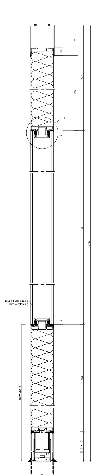
Trennwand mit Verglassung Wall with Window
