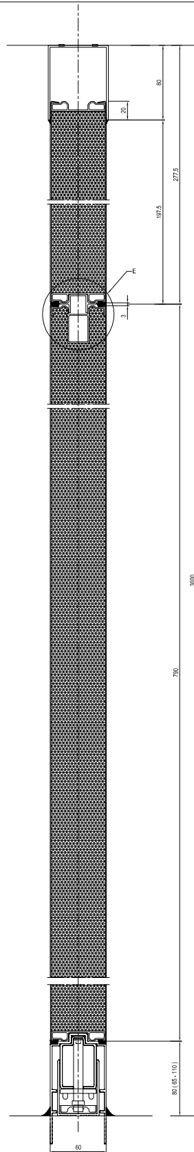
Trennwand mit Polyurethan Kern Wall with polyurethane core
